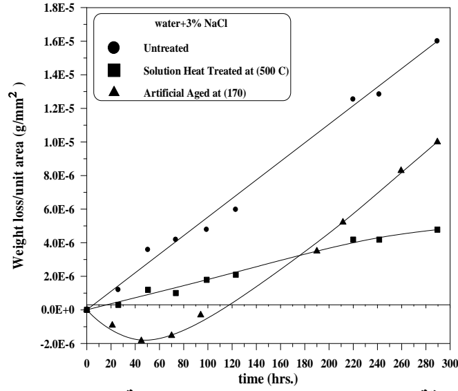
الشكل (1) العلاقة بين الوزن المفقود لوحد المساحة وزمن التعرض للوسط التآكلي (3wt%NaCl)
